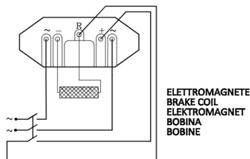
FRENATA RAPIDA - QUICK BRAKING - SCHNELL BREMSVORGANG FRENADA RAPIDA - FREINAGE RAPIDE
