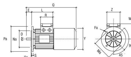
BM B14
