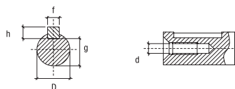
Estremità d'albero
