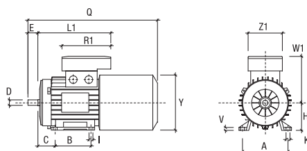
BM 160÷225 B3
