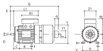
BAE B5
