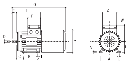
BM B5
