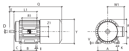
BM 160÷225 B3
