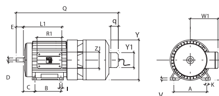
Estremità d'albero
