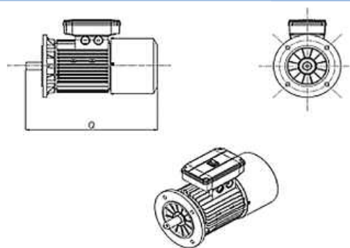
Serie BMAV
