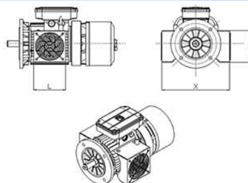
Serie BASV
