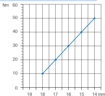
BA 100
