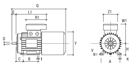
160÷225 B3
