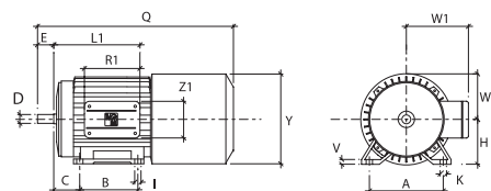
160÷225 B3
