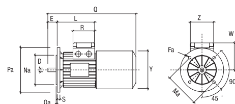
B14
