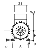
BAE B5
